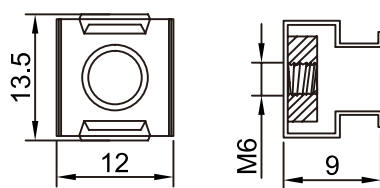
Cage Nut
